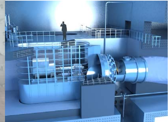
Site : GANGCHUN SHP Head : 4.7m Flow : 44cms Output : 1740kW x 3unit Speed : 116 rpm
